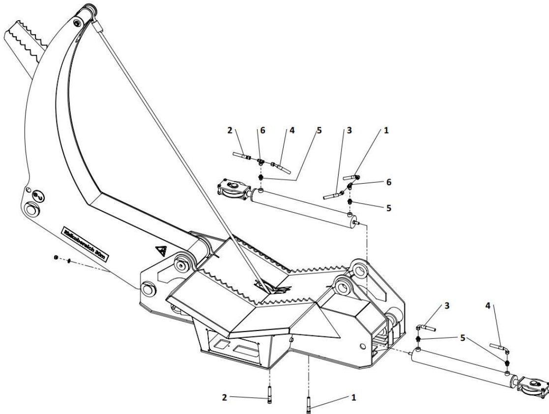
Hydraulik - Schläuche und Verschraubungen - Artikel-Nummer hydraulic hoses and fittings - part-no.
