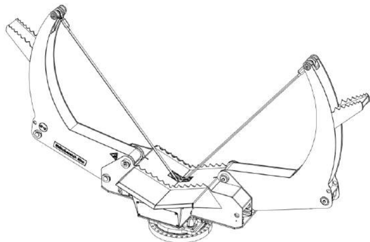
dargestellt im Bild „verstärkte Version“ des Dreh-& Kiplagers
